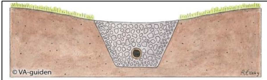
Figur 10-8. Princip för krossdike. (VA-Guiden, u.å.)
