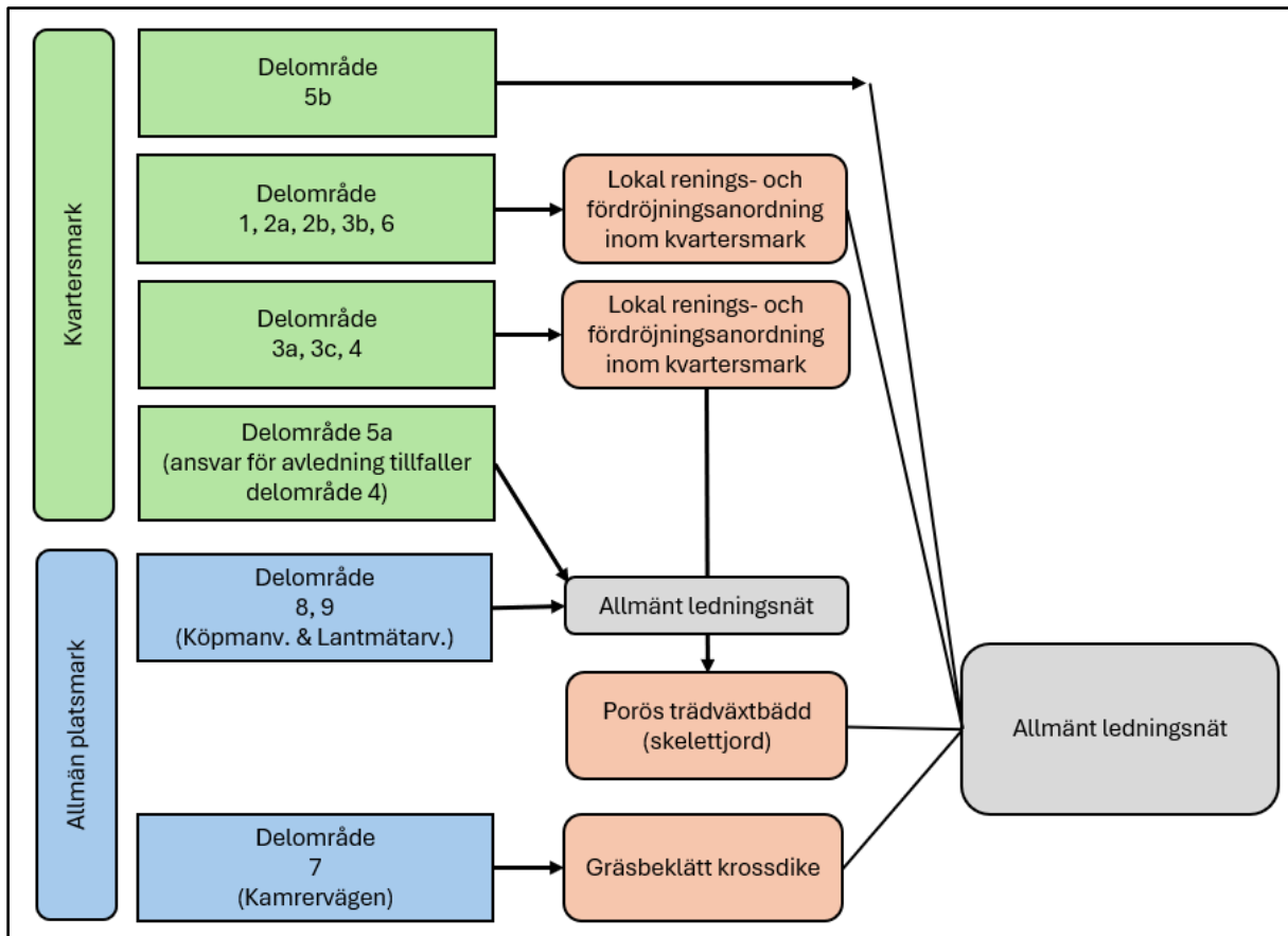
Figur 10-14. Sammanfattande flödesschema över föreslagen systemlösning utifrån tekniska delavrinningsområden, planerad situation.
