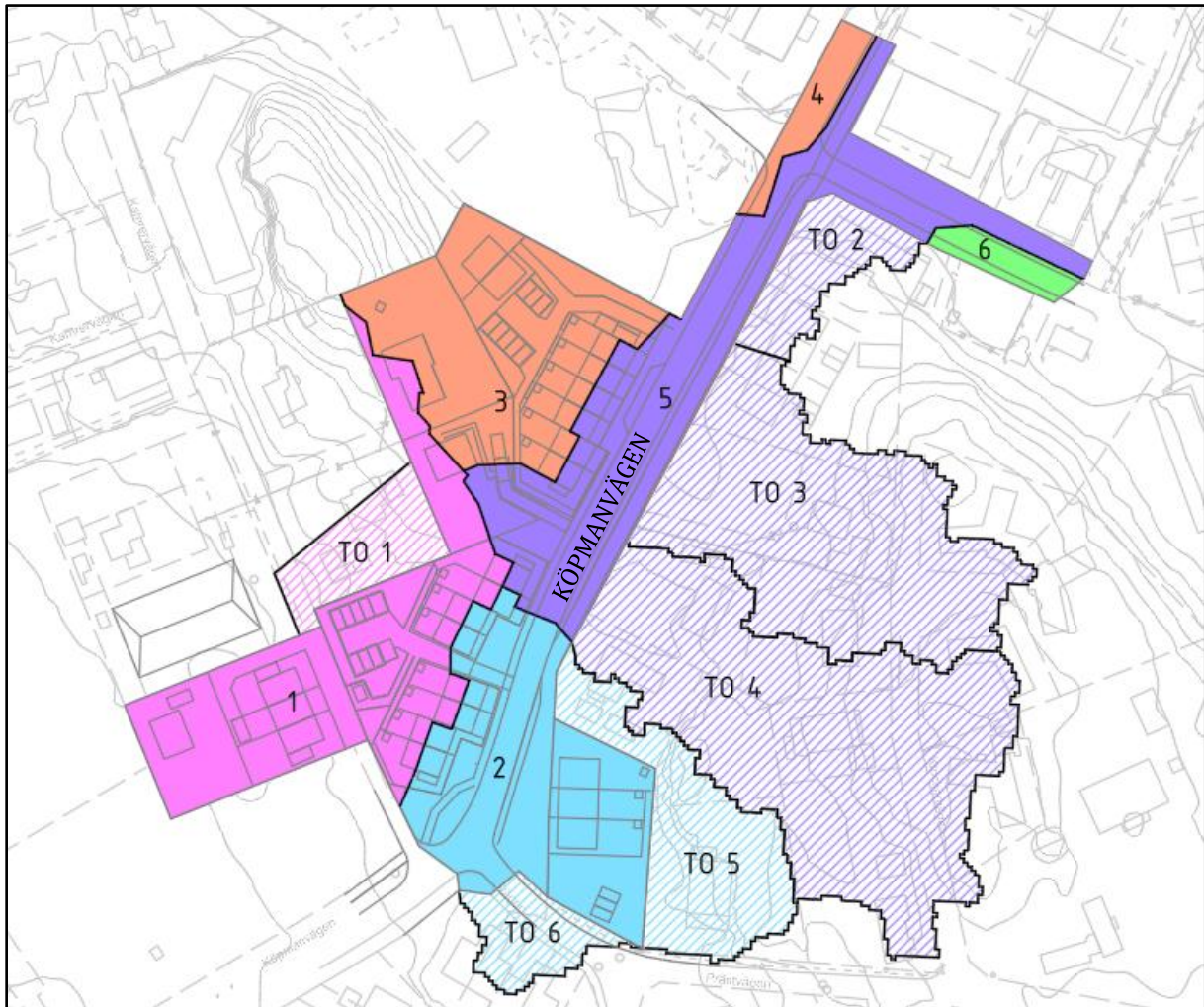
Figur 7-3. Indelning av topografiska delavrinningsområden, planerad situation. Svarta linjer illustrerar vattendelare.
