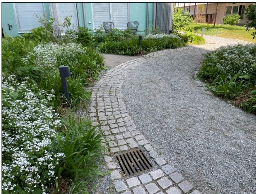
Figur 10-1. Exempel på utformning med genomsläppliga beläggning inom gårdsmark. (Marktema, 2025)
