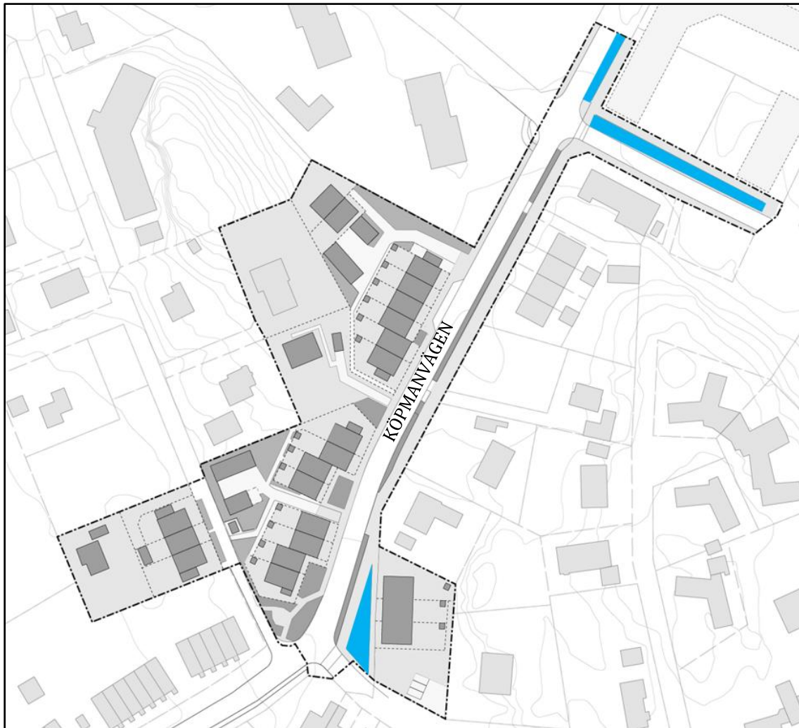
Figur 10-10. Översikt visande förslag på ytor (blå) för dagvattenhantering av Köpmanvägen och Lantmätarvägen. (Bearbetad från: Landskapslaget, 2025-11-14)
