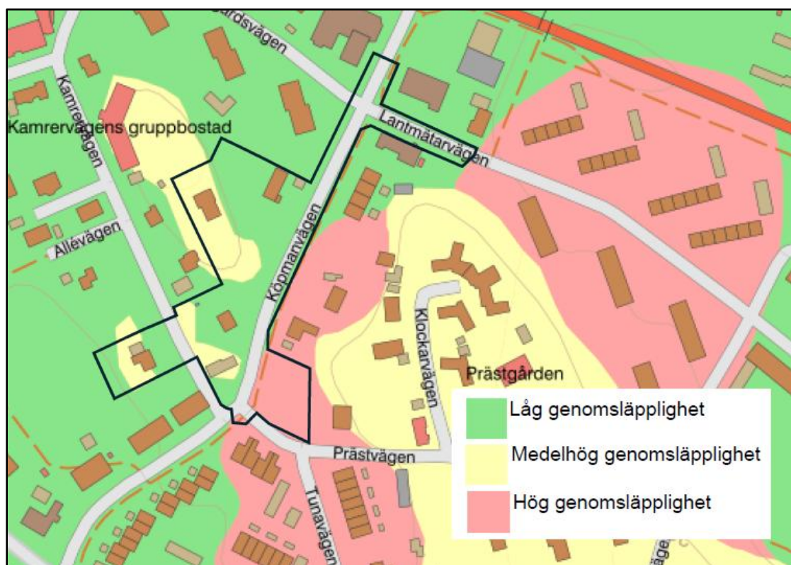
Figur 6-3. Översikt visande att partier av medelhög och hög genomsläpplighet kan antas förekomma, men att genomsläppligheten främst kan förväntas vara låg. Planområdets ungefärliga utbredning illustreras med svart linje. (SGU, u.å.)
