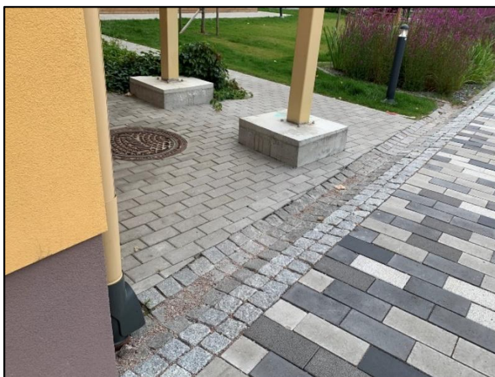
Figur 10-6. Exempel på takavvattning via öppna utkastare och rännalar. (Marktema, 2025)
