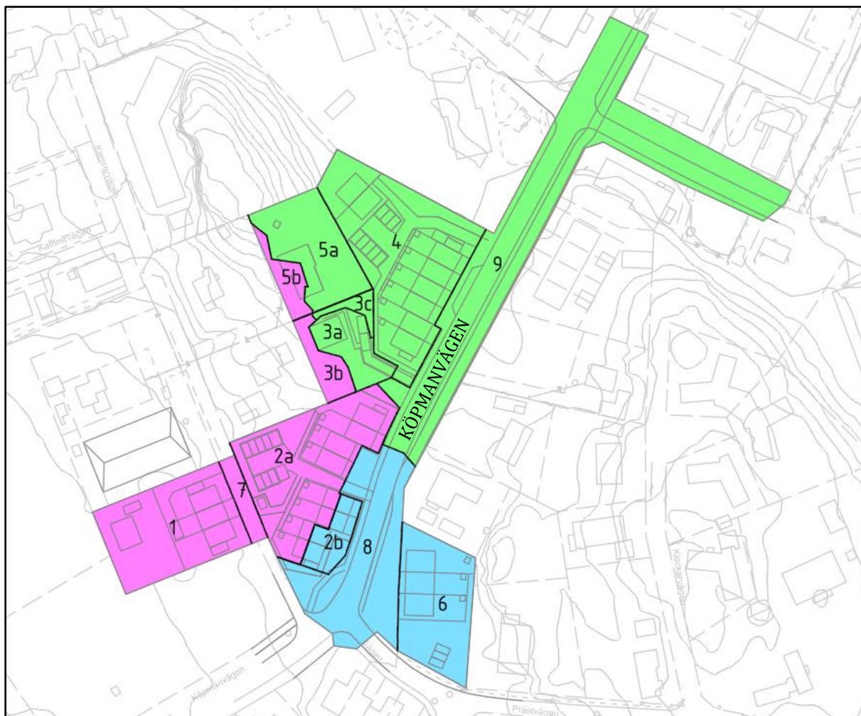
Figur 7-4. Indelning av tekniska delavrinningsområden, planerad situation. Svarta linjer illustrerar tekniska vattendelare.
