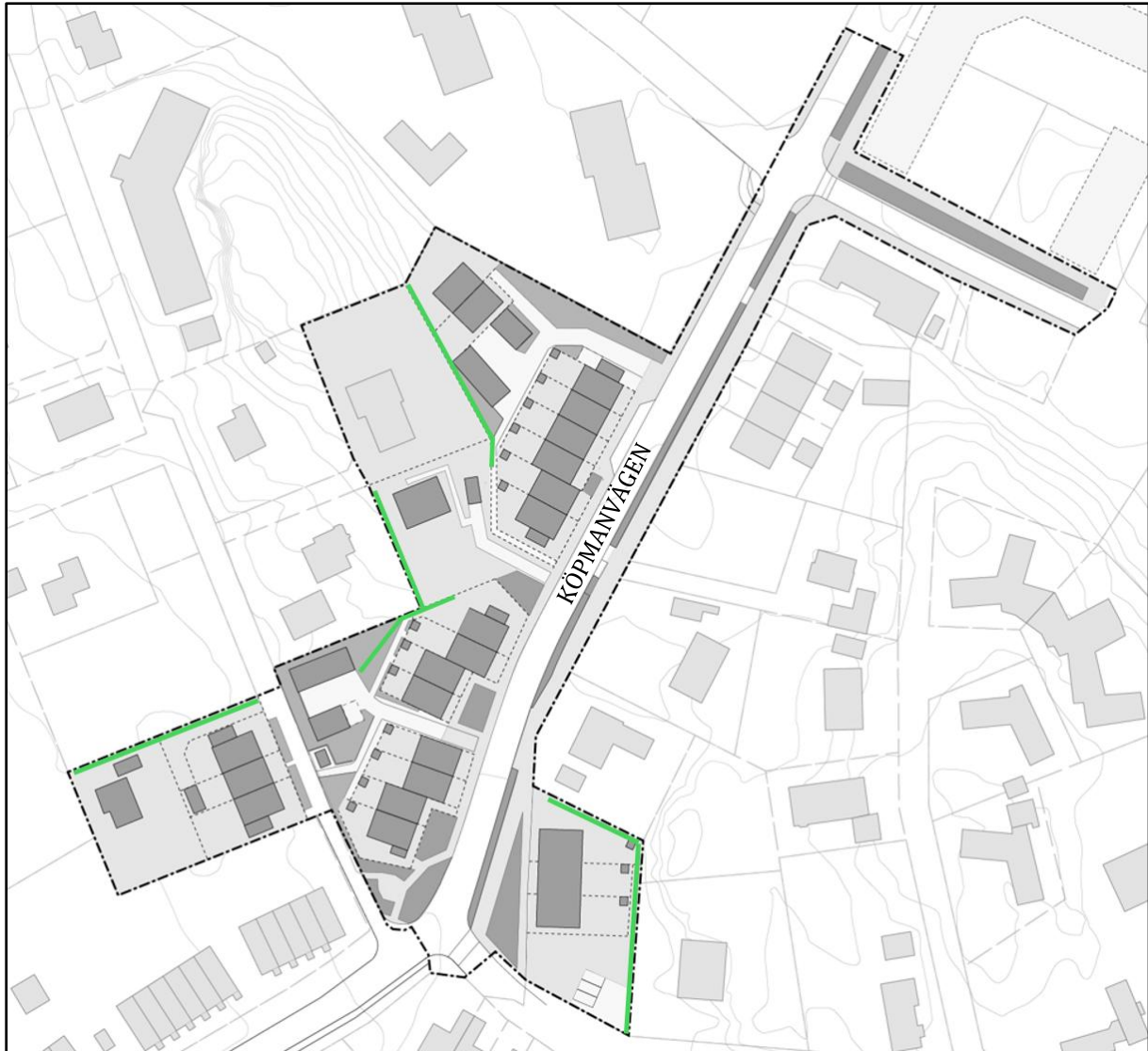
Figur 10-15. Översikt visande förslag på placering av avskärande diken (gröna linjer) för avledning av diffus tillrinning. (Bearbetad från: Landskapslaget, 2025-11-14)
