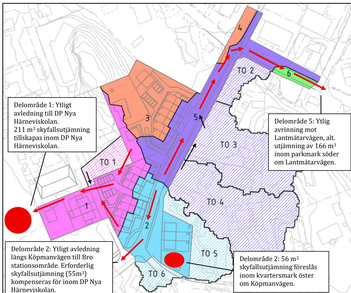
Figur 11-3. Schematisk illustration av beskrivna specifika översvämningsåtgärder för delområde 1, 2 och 5. Röda pilar illustrerar sekundär avledning och röda cirklar illustrerar lägesförslag för översvämningsytor.
