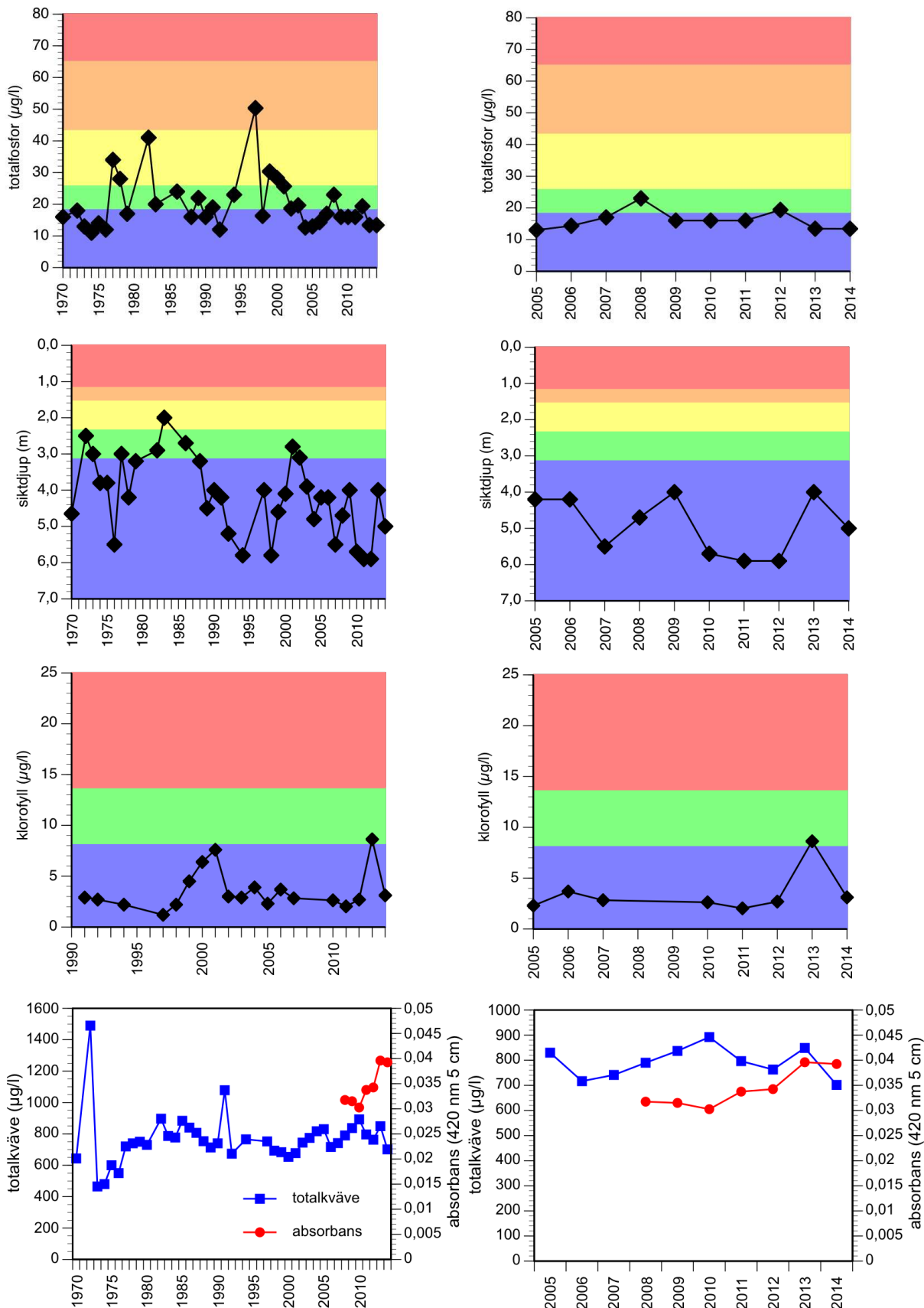
Figurerna ovan visar ekologisk status avseende fysikalisk-kemiska kvalitetsfaktorer (näringsämnen/totalfosfor, ljusförhållanden/siktdjup) och biologiska kvalitetsfaktorer (klorofyll). Färgerna motsvarar intervall för respektive statusklass (blå – hög, grön – god, gul – måttlig, orange – otillfredsställande, röd – dålig). Dessutom visas
