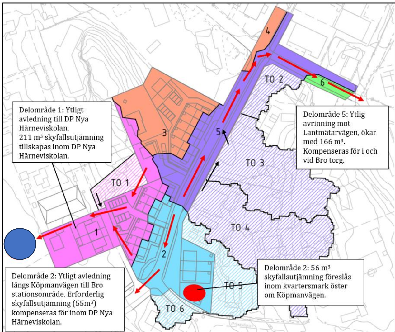
Figur 30. Flödesriktningar efter exploatering samt principiellt förslag till placering av översvåmningsytor inom planområdet (röd yta). Kompletterande yta utom planområdet redovisas med blå cirkel. Bild Marktema, justerat avseende delområde 5.
