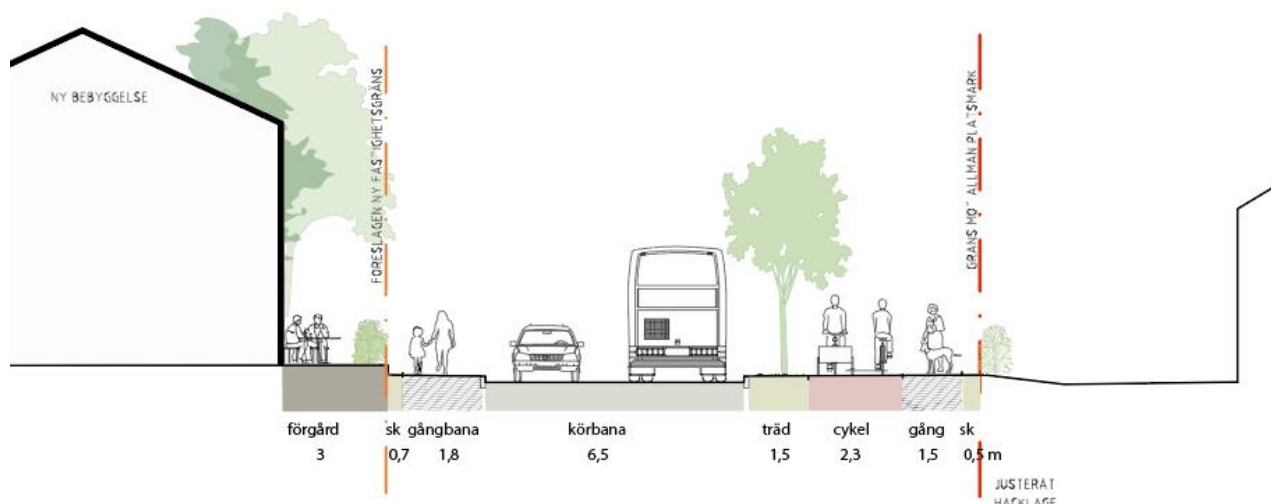
Figur 22. Principsektion för ny utformning av Köpmanvägen, med ny gångbana på den västra sidan av gatan och en breddad gång- och cykelbana på den östra sidan. "Sk" avser skyddsremsa, vilket avser en yta med genomsläpplig beläggning som kan fungera för tex snöupplag och belysningsarmaturer i gräns mellan gata och tomtmark.
