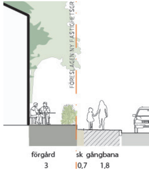
Principsektion för upphöjd förgårdsmark med avskärmade plantering längs gångbana.
