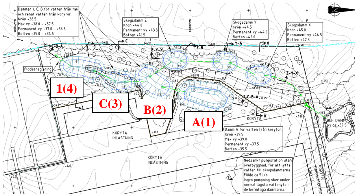
Figur 6. Förprojektering av nya dagvattendammar inom detaljplanens västra delar. Numrering inom parentes "( )" avser dagvattendammarnas benämning i upprättad dagvattenutredning (Sweco, 2024). (modifierad från VAP VA-projekt, 2022).
